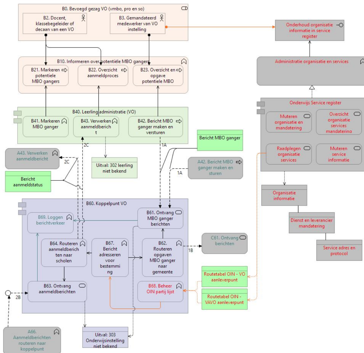
Figuur 10: Architectuurplaat van het vo-koppelpunt (paars) en context: gekoppelde leerlingadministraties (groen) die de bedrijfsprocessen en daarmee gebruikers (oranje) ondersteunen. In grijs, buiten scope van dit project, rechts het onderwijs service register en aan de linkerkant de verwerking van rapportages.
