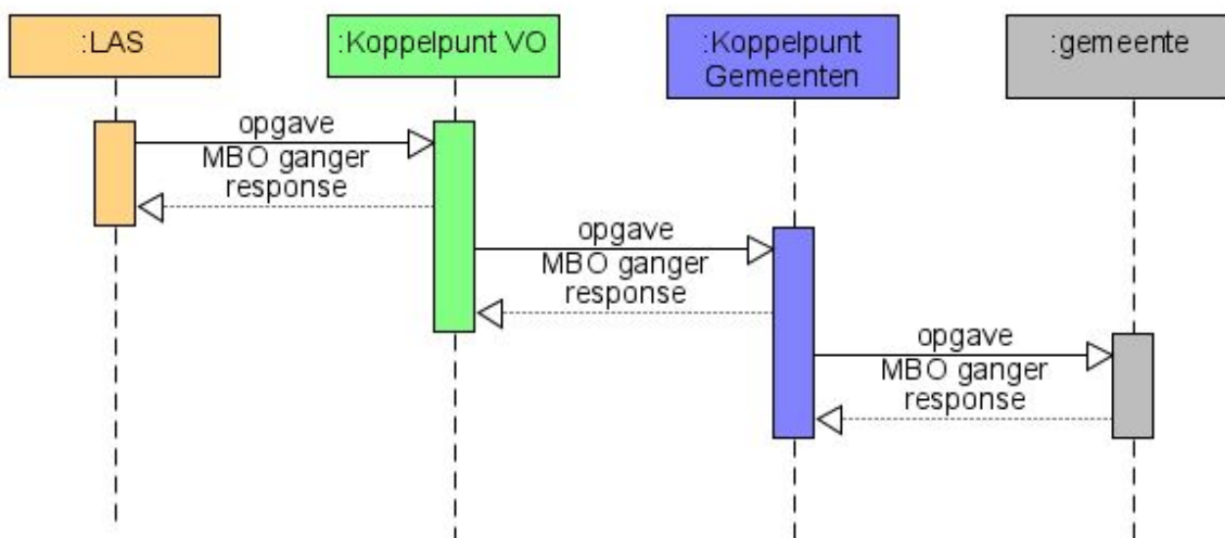
Figuur 9: Illustratie van de sequentie van aanroepen en responses tussen afzender en ontvanger in het geval van een opgave mbo gangster. Hierin wordt weergegeven dat een ontvanger van een bericht de eigen controles uitvoert en een respons geeft aan de afzender, en het bericht daarna pas doorstuurt naar de volgende partij. Afhandeling van aanmeldberichten zal op analoge wijze plaatsvinden.
