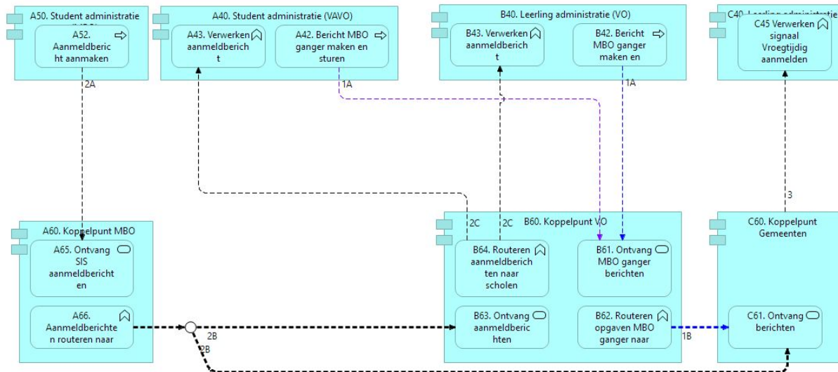
Figuur 8: Overzicht van de berichtstromen en bijbehorende technische interfaces. Berichtstroom 1 geeft opgave mbo ganger weer, berichtstroom 2 geeft het aanmeldbericht bestemd voor onderwijsinstellingen weer. Berichtstroom 3 tussen koppelpunt gemeenten en de gemeenten wordt ingericht volgens de conventies van de gemeenten.
