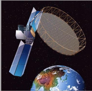
SIGINT satellites
